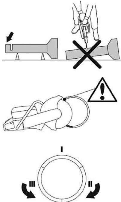
Рис. 15 Резка труб
